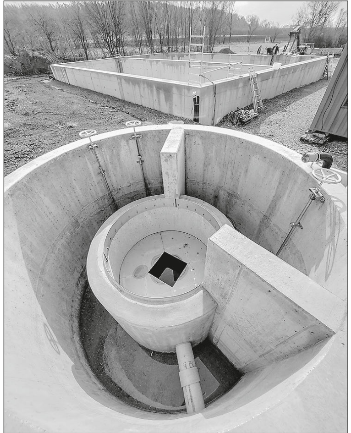
Vorne: Verteilbauwerk, im Hintergrund das neue Belebungsbecken
